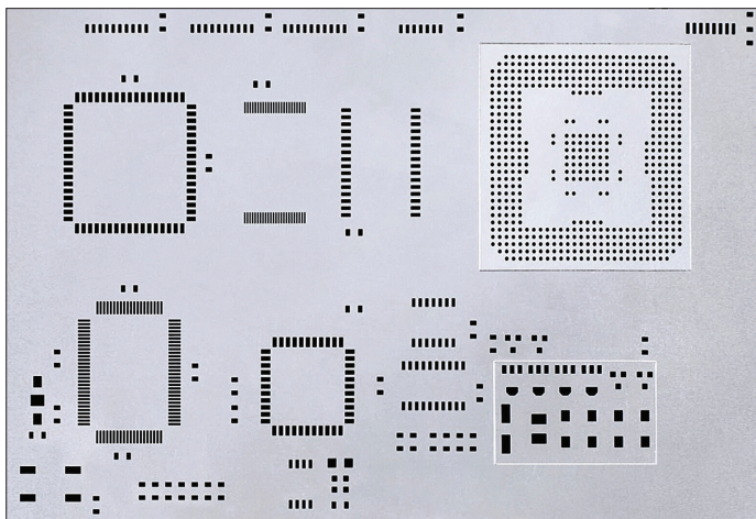
Многоуровневый трафарет (StepUp/StepDown)
